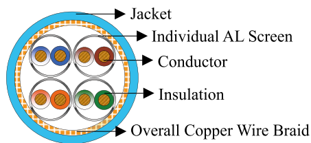
Cat6A S/FTP
